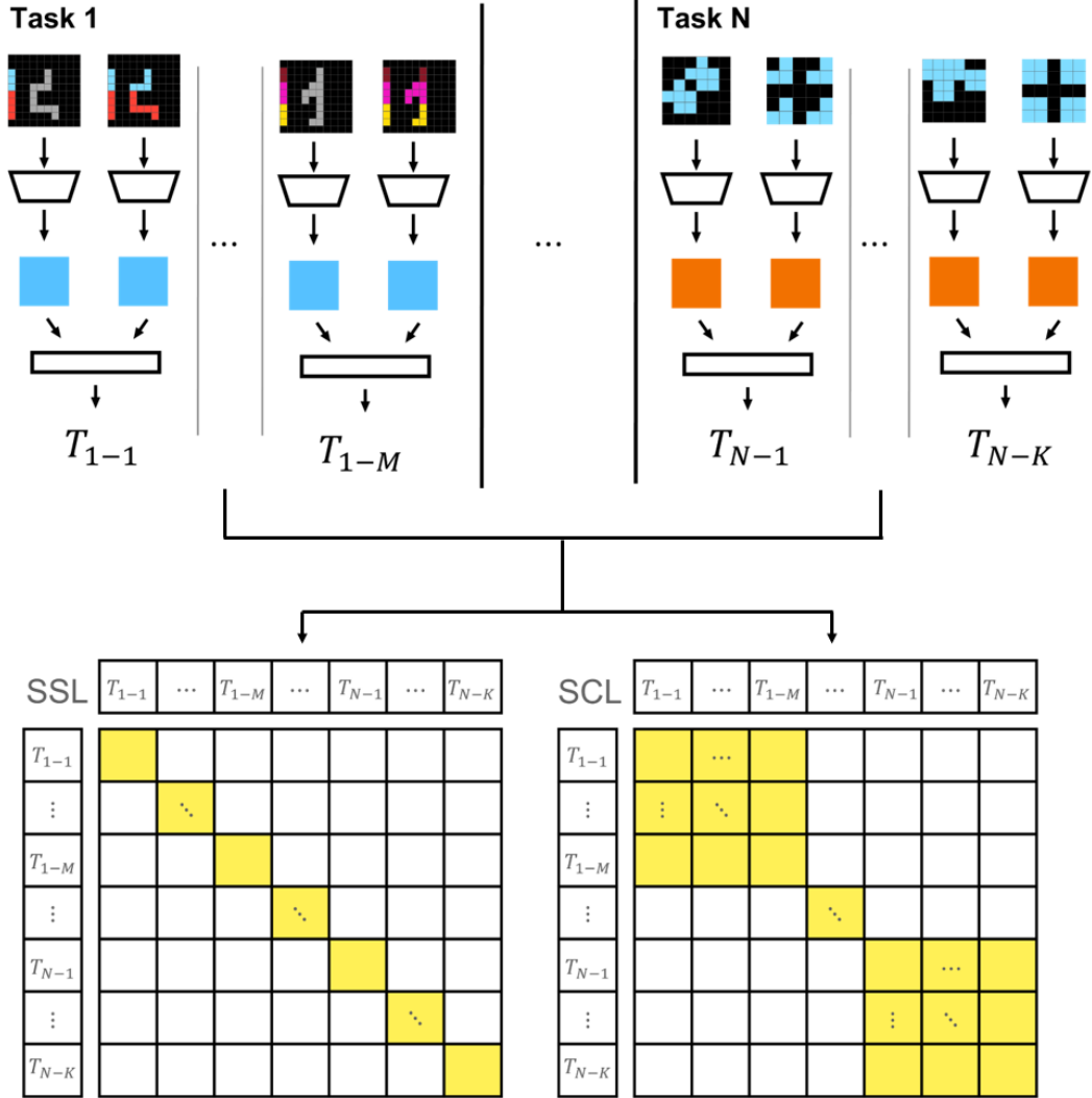
Figure 2.2: 각각의 문제를 나타내는 표현 벡터를 활용해 대조 학습을 진행하는 그림. 그림에서 T_{N-K} 는 N 번째 문제의 K 번째 입력-출력 쌍을 나타내는 표현 벡터이다.
