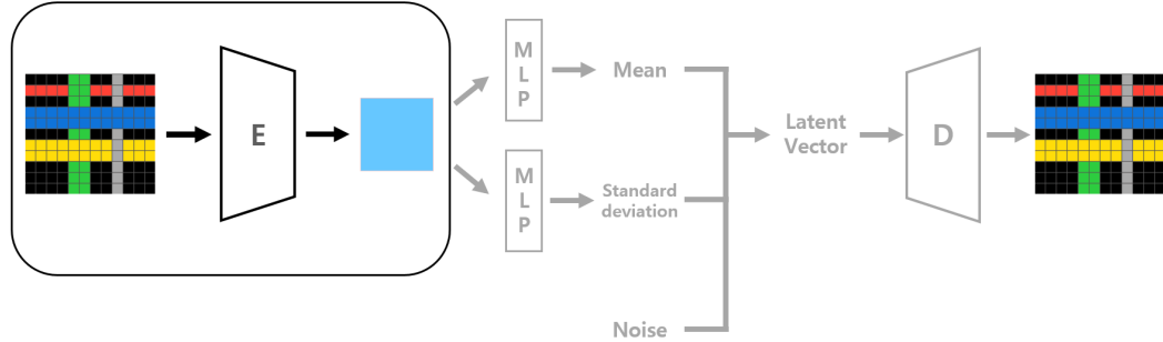
Figure 2.3: VAE 구조. 인코더에서 입력 데이터를 압축하는 과정을 거치고 압축된 정보에 평균과 표준편차를 표현하는 값을 파라미터를 통해 출력한다. 그리고 예측한 표준편차에 가우시안 노이즈를 곱한 후, 평균을 더해 표현 벡터를 생성한다.
