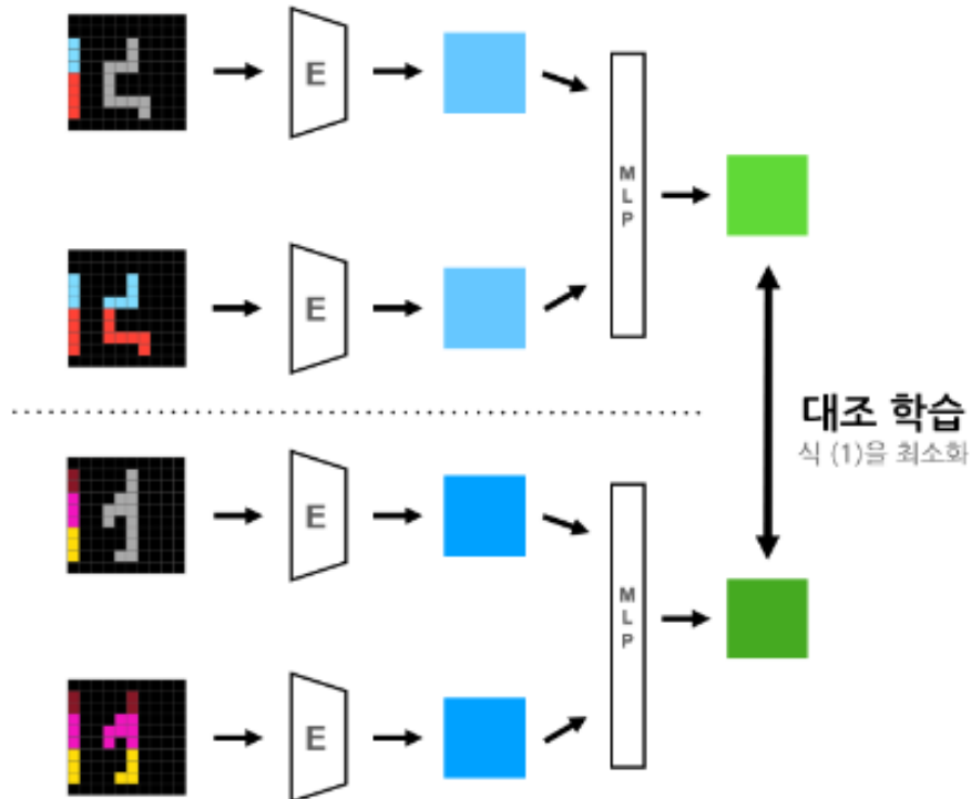
Figure 2.1: ARC 문제의 입력-출력 쌍에 대해 표현 벡터를 추출하고 대조 학습을 하는 과정을 나타낸 간단한 모식도.
