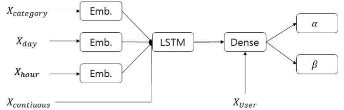
그림 2 WTTE-RNN을 참고한 Model
